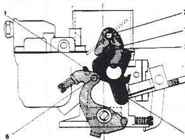
Fig. II. Ralenti accéléré - Warmlauf - Fast idle
