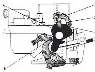
Fig. III. Ralenti normal - Normal Leerlauf - Normal idling
