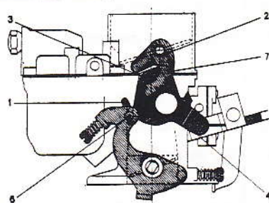
Fig. I. Départ à froid - Kaltstart - Starting from cold
