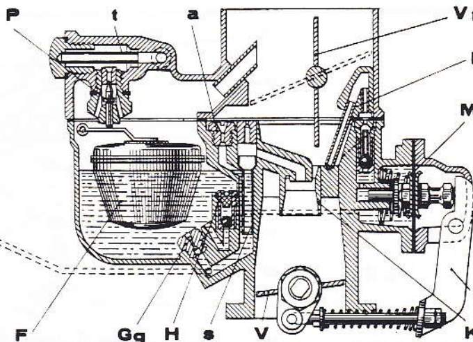
Fig. II. Ralenti accéléré - Warmlauf - Fast idle
