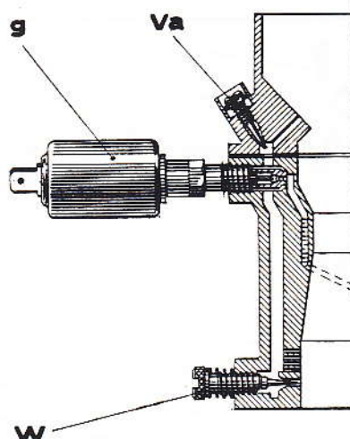
Fig. I. Départ à froid - Kaltstart - Starting from cold
